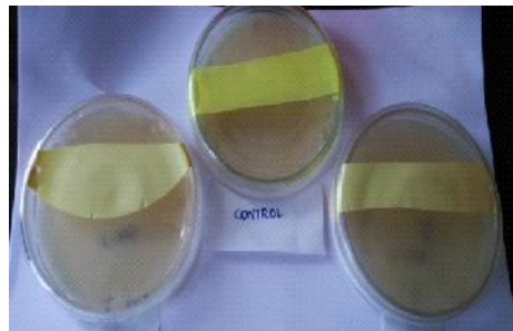
HCN production
